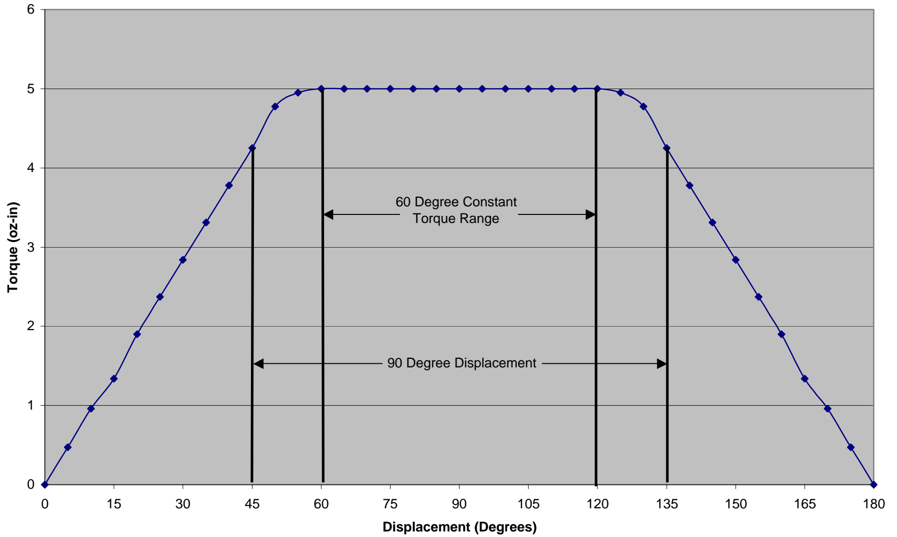
TMR-060-005-2H Torque vs. Displacement
